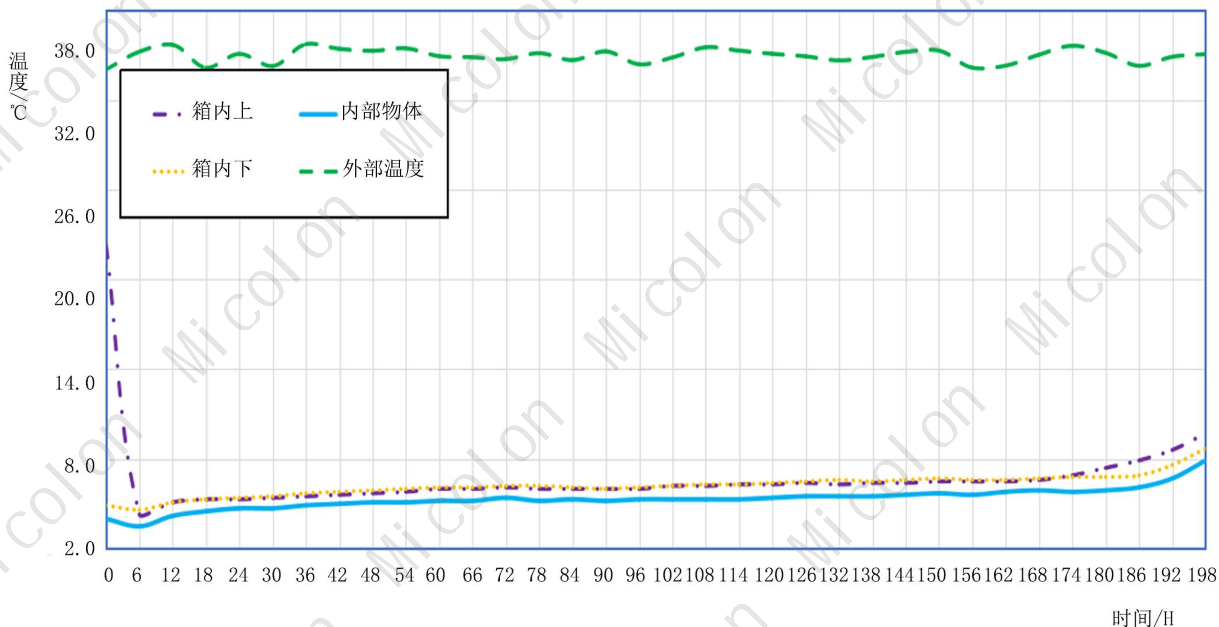
2°C~8°C温度曲线(PCM)
